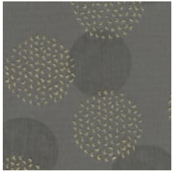
Orb-Mercury
