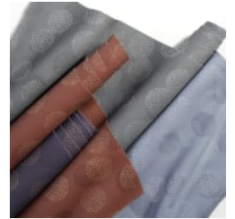
Orb-Mars
